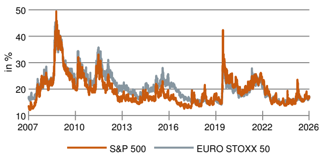
Volatilitätsentwicklung* – Langfristig
